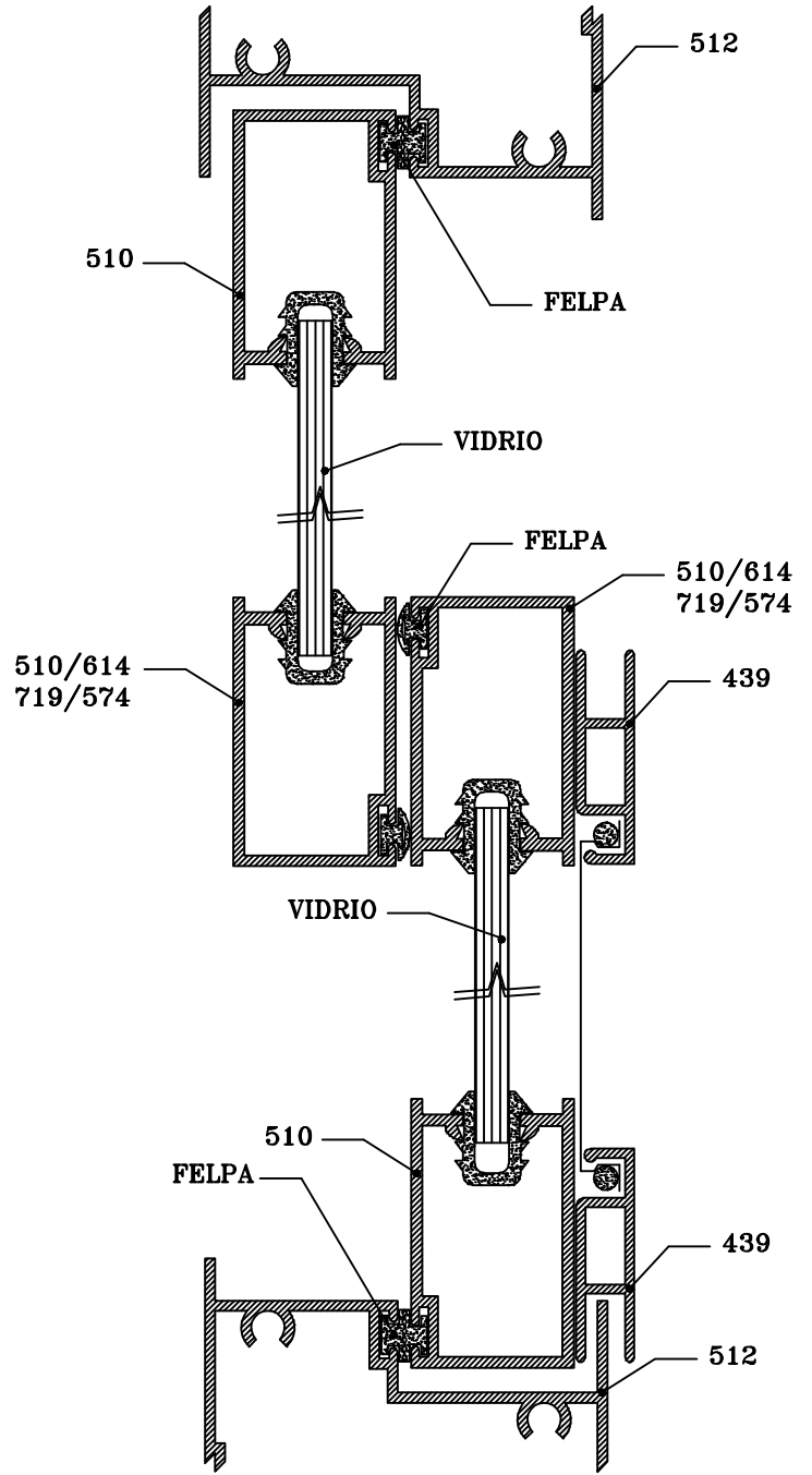
CORTE HORIZONTAL
