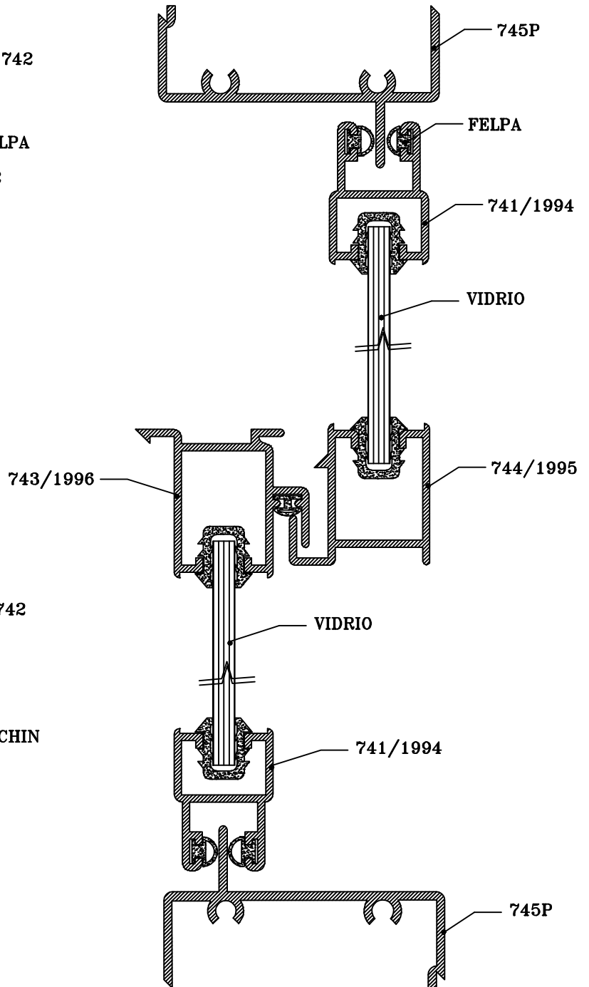
CORTE HORIZONTAL
