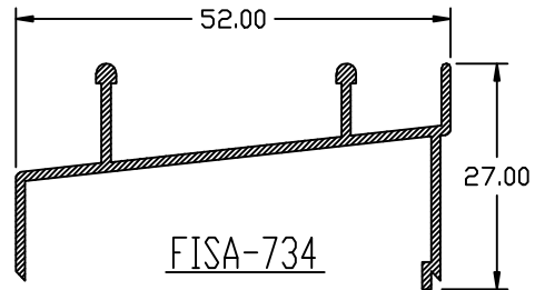
RIEL INFERIOR
