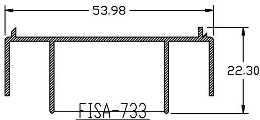
RIEL SUPERIOR
