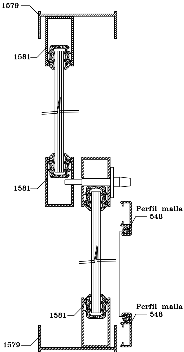
CORTE HORIZONTAL
