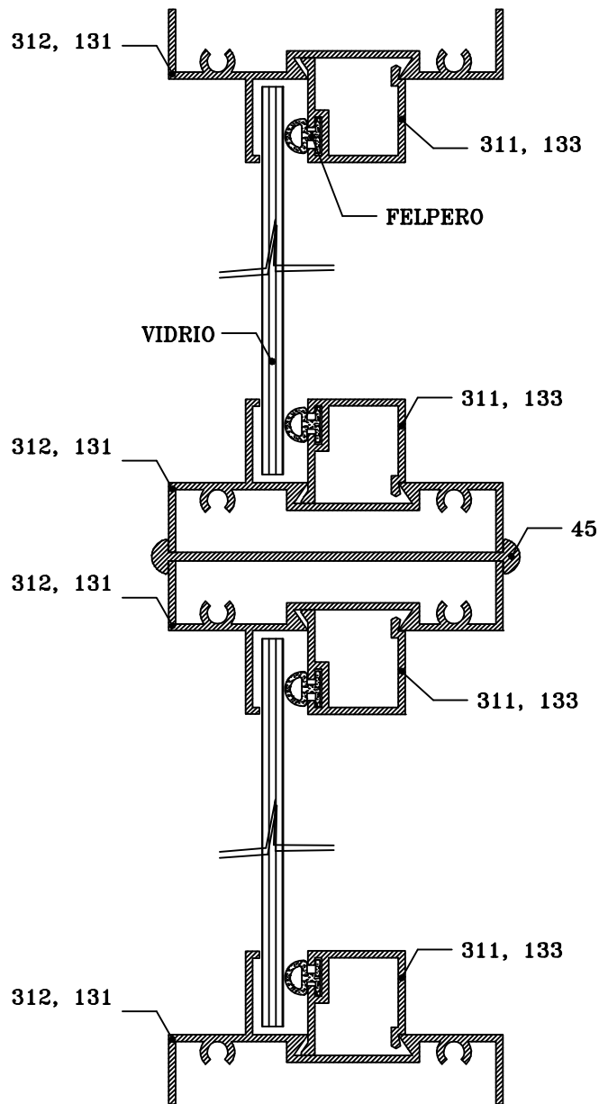
CORTE HORIZONTAL
