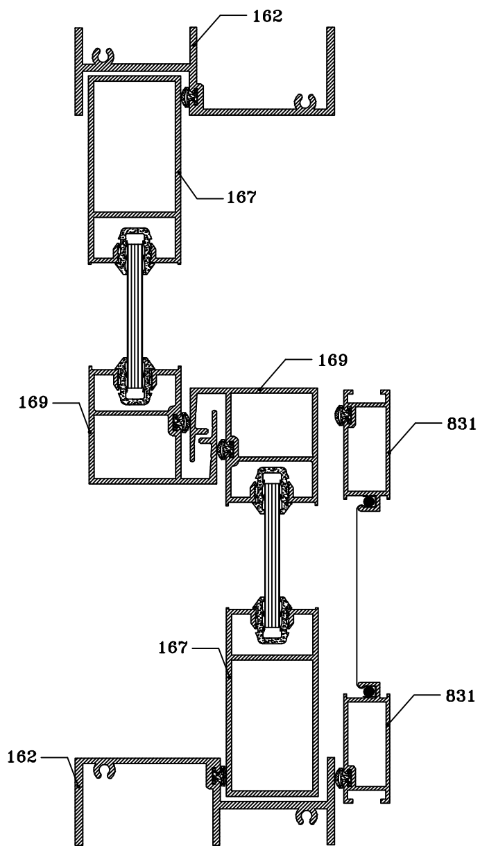
CORTE HORIZONTAL
